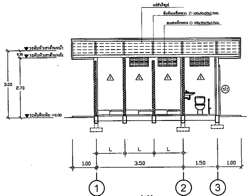
รูปตัด B
