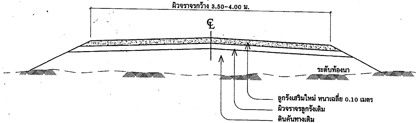
รูปตัดขวางแสดงโครงสร้างถนน และ คุณสมบัติวัสดุ มาตรฐาน NOSCALE
