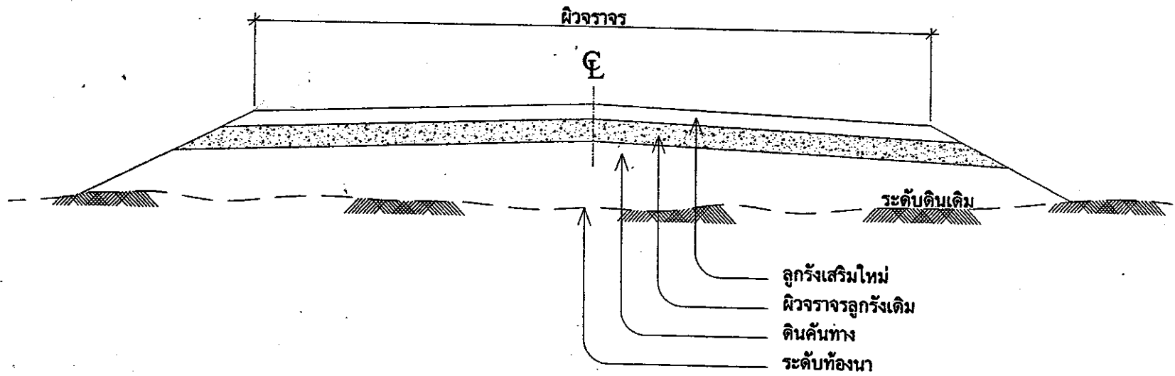
รูปตัดขวางแสดงโครงสร้างถนน และ คุณสมบัติวัสดุ มาตรฐาน NOSCALE
